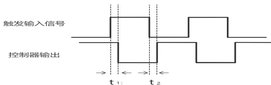
图 8 常亮模式时序图
