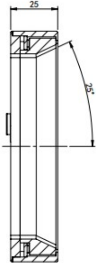
剖面 A-A
