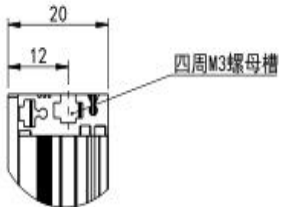
局部视图 A 比例 1 : 1
