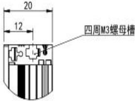
局部视图 A 比例 1 : 1
