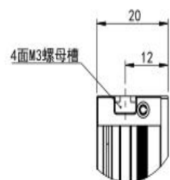
局部视图 A 比例 1 : 1
