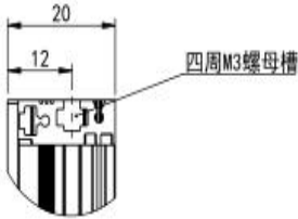
局部视图 A 比例 1 : 1
