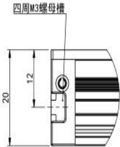
局部视图 A 比例 3 : 2
