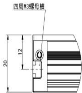
局部视图 A 比例 3 : 2
