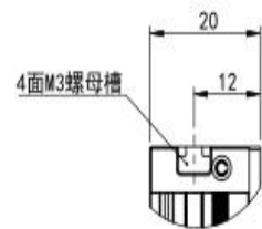
局部视图 A 比例 1 : 1
