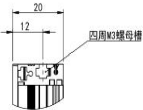
局部视图 A 比例 1 : 1
