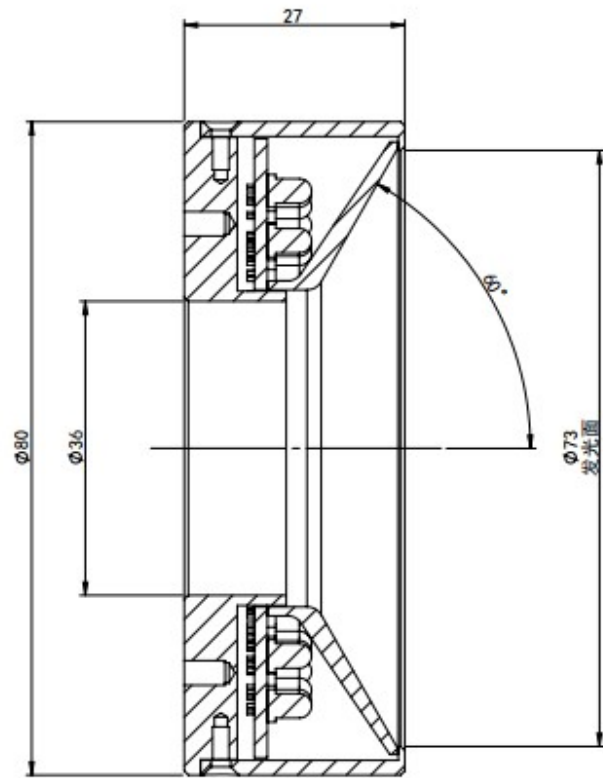
剖面 A-A
