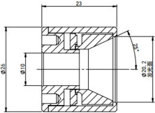
剖面 A-A
