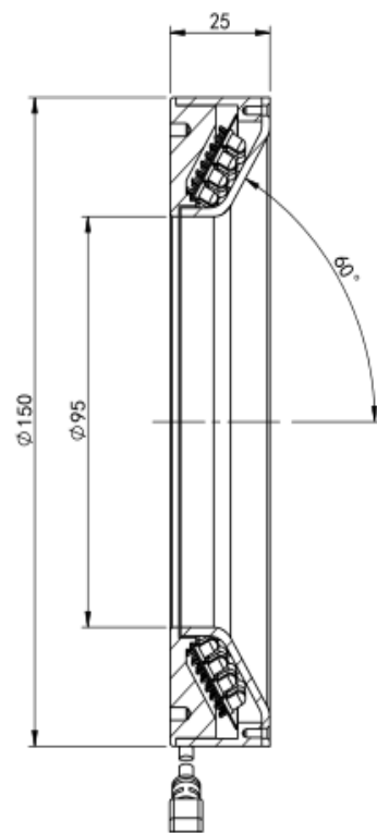
剖面 A-A
